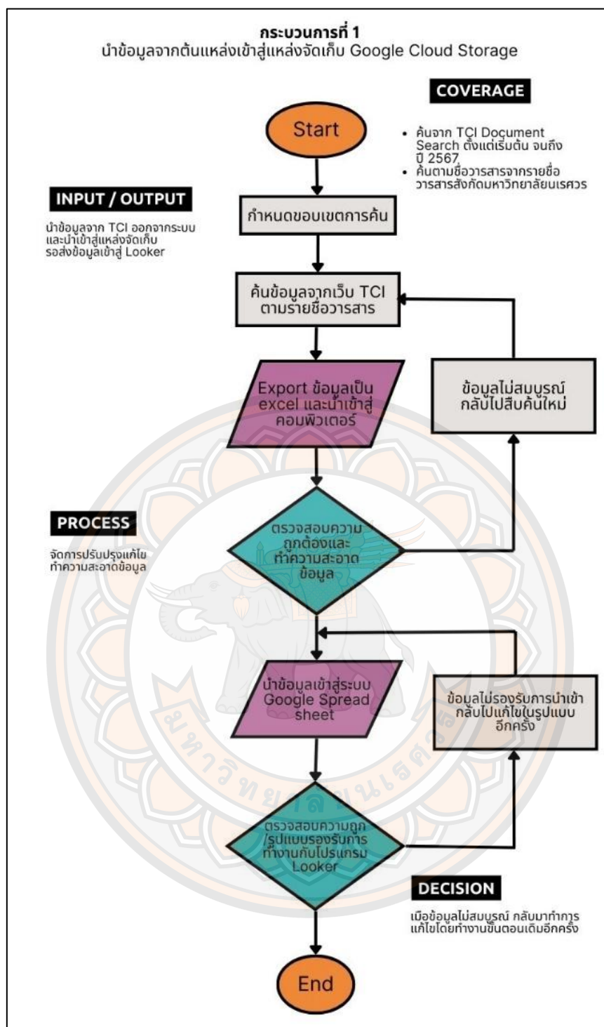
ภาพที่ 7 แสดงกระบวนการนำข้อมูลเข้าแหล่งจัดเก็บบน Cloud Storage
