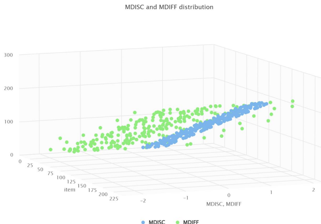
ภาพที่ 59 แสดงการกระจายระหว่างค่าความยากแบบพหุมิติของข้อสอบ กับค่าอำนาจจำแนกแบบพหุมิติของข้อสอบ
