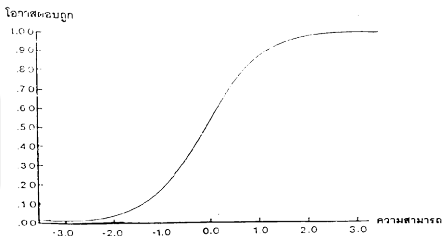
ภาพที่ 2 โค้งแสดงลักษณะของข้อสอบตามโมเดลโลจิสติกแบบ 1 พารามิเตอร์
