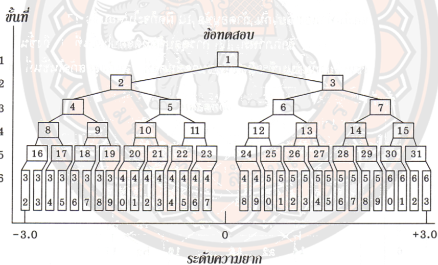
ภาพที่ 12 โครงสร้างของแบบทดสอบรูปพีระมิดแบบโรบินส์มอนโร
