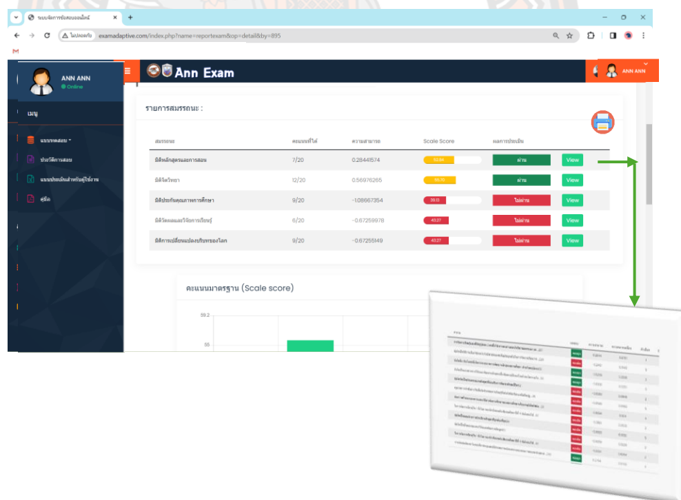
ภาพที่ 15 หน้าจอแสดงผลการวิเคราะห์ความสามารถของผู้สอบ Theta ( \theta ) , ค่า Scale Score และผลการประเมินแยกตามมิติ
