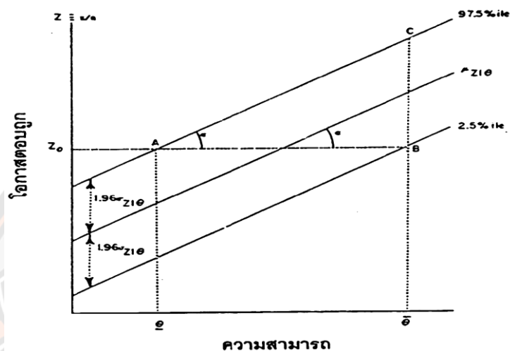
ภาพที่ 5 ช่วงแห่งความเชื่อมั่นแอสิมโทติก 95% ( \theta_{\underline{}} , \theta_{\overline{}} ) สำหรับความสามารถ \theta
