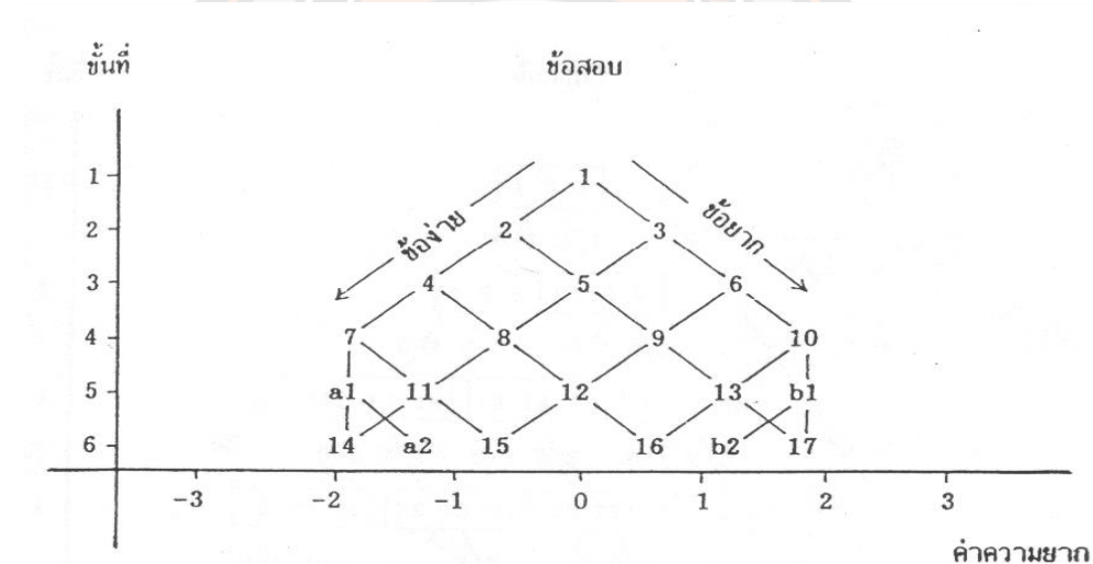
ภาพที่ 14 โครงสร้างของแบบทดสอบรูปพีระมิดแบบรักษาการสะท้อนกลับ
