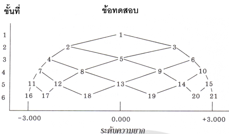
ภาพที่ 11 โครงสร้างของแบบทดสอบรูปพีระมิดขนาดชั้นแปด
