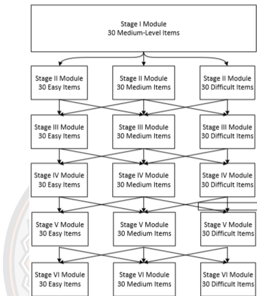
ภาพที่ 18 ตัวอย่างขั้นตอนและกฎเส้นทางของ MST ที่มา: Brossman and Guille (2014)
