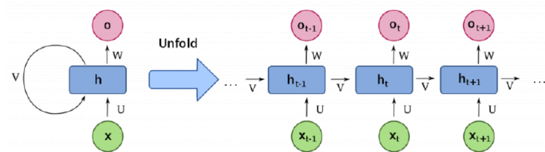
ภาพที่ 28 โครงสร้างของโครงข่ายประสาทเทียมแบบวนกลับ
