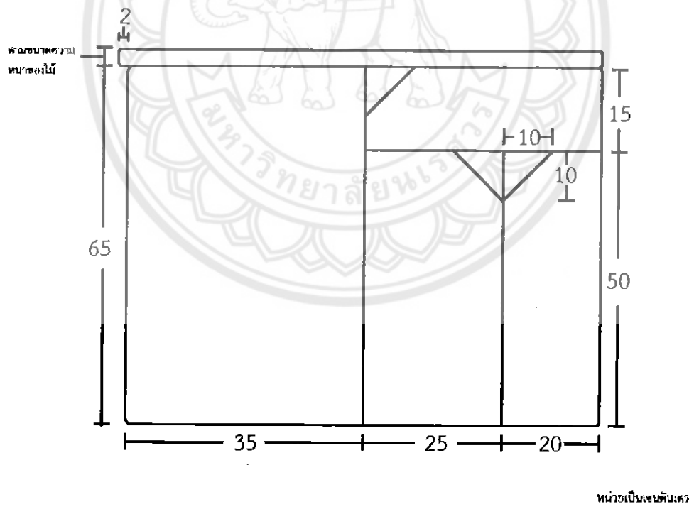
ภาพที่ 4.14 ภาพ Dimension ด้าน Front ของ โตะ
