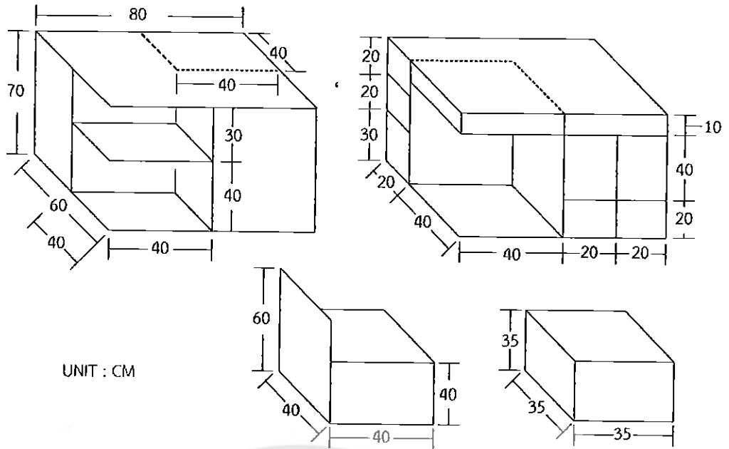
ภาพ 4.3 ภาพการออกแบบขนาดของ โต๊ะอาหาร ไม้ยางพาราสำหรับใช้ในหอพัก
