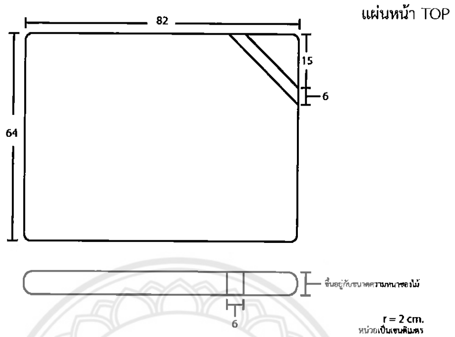
ภาพที่ 4.13 ภาพ Dimension ด้าน Top ของ โตะ
