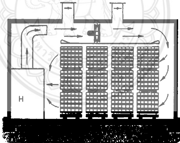
ภาพที่ 2.11 ภาพการอบไม้ยางพาราแปรรูป ที่มา: http://www.thesolardryer.com/ เข้าถึงได้จาก http://www.thesolardryer.com/su/drying/solardry-thai.htm
