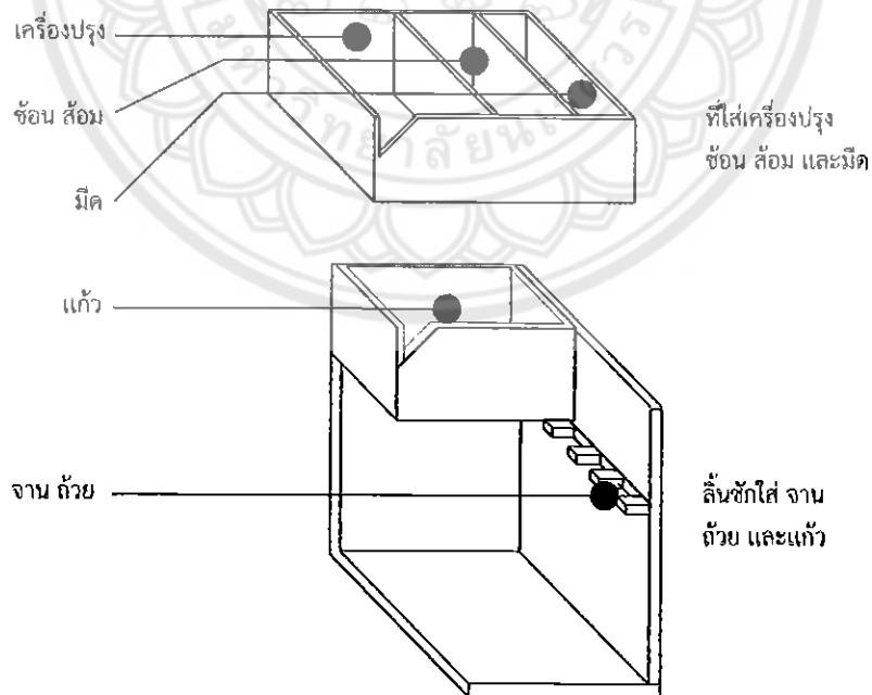
ภาพที่ 4.10 ภาพ Perspective ของการจัดพื้นที่อุปกรณ์ที่เก็บในลิ้นชัก
