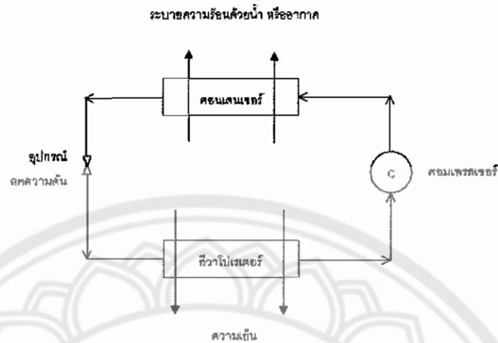
รูปที่ 2.2 วงจรทำความเย็น
