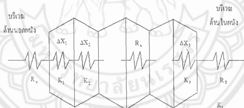
รูปที่ 2.2 แสดงภาพการถ่ายเทความร้อนผ่านผนังอาคาร แบบมีช่องว่างอากาศอยู่ตรงกลาง
