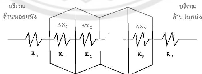
รูปที่ 2.1 แสดงภาพการถ่ายเทความร้อนผ่านผนังอาคาร
