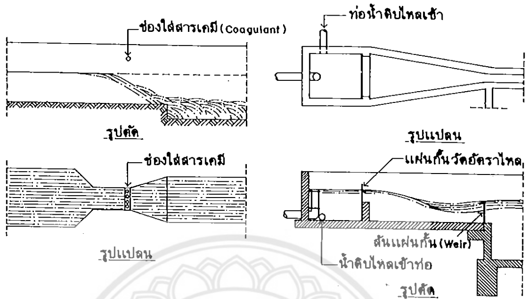
รูปที่ 2.5 ระบบถังกวนเร็วแบบต่าง ๆ
