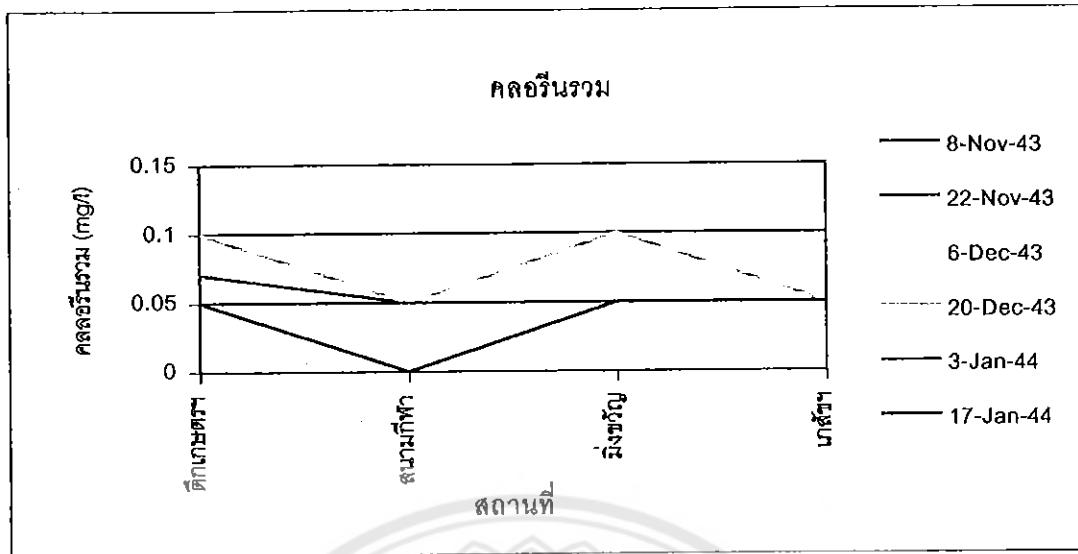
รูปที่ 4.11 คลอรีนรวมในเส้นท่อน้ำประปาที่ 2
