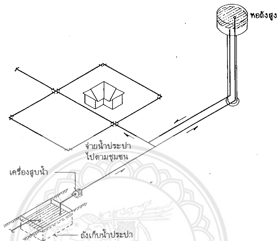
รูปที่ 2.16 ระบบแจกจ่ายน้ำประปาด้วยวิธีสูบจ่ายร่วมกับหอถังสูง ที่มา ดร.เกรียงศักดิ์ อุดมสิน โรจน์, 2539
