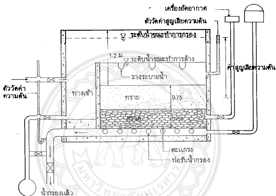
รูปที่ 2.10 แสดงเครื่องกรองความดัน ที่มา ดร.เกรียงศักดิ์ อุดมสินโรจน์, 2539
