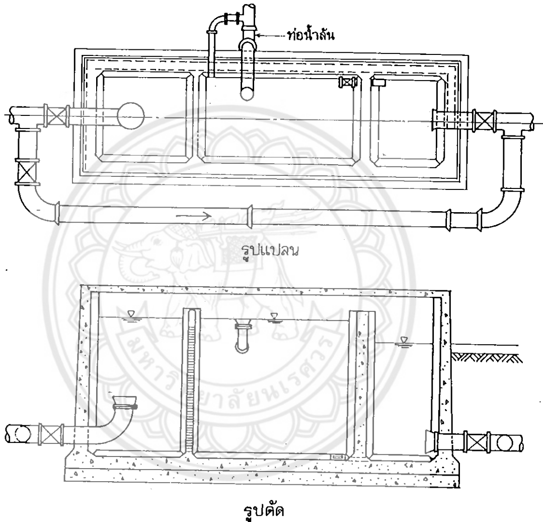
รูปที่ 2.17 แสดงถังเก็บน้ำบนพื้นดิน ที่มา ดร.เกรียงศักดิ์ อุคมสิน โรจน์, 2539
