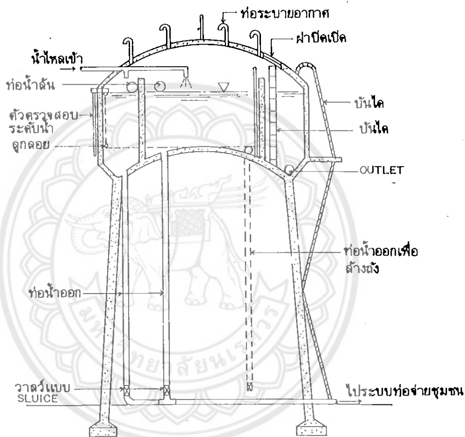
รูปที่ 2.18 หอดังสูง
