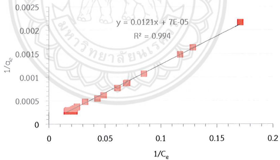
รูปที่ ๓.4 แสดงผลของสมการไอโซเทอรั่มแลงมัวร์ของขนาดของตัวดูดซับ 40 mesh ความสูงของตัวดูดซับ 5 เซนติเมตร อัตราการไหล 5 มิลลิลิตรต่อนาที และความเข้มข้นเริ่มต้นของสารละลายสีย้อมเมทิลีนบลู 50 มิลลิกรัมต่อลิตร
