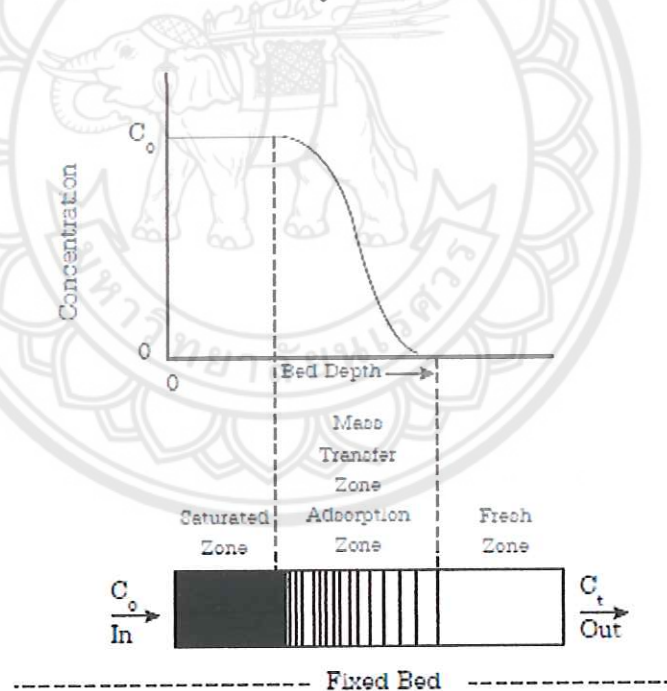
รูปที่ 2.1 แสดงความเข้มข้นภายในคอลัมน์ของสารดูดซับ [2]
