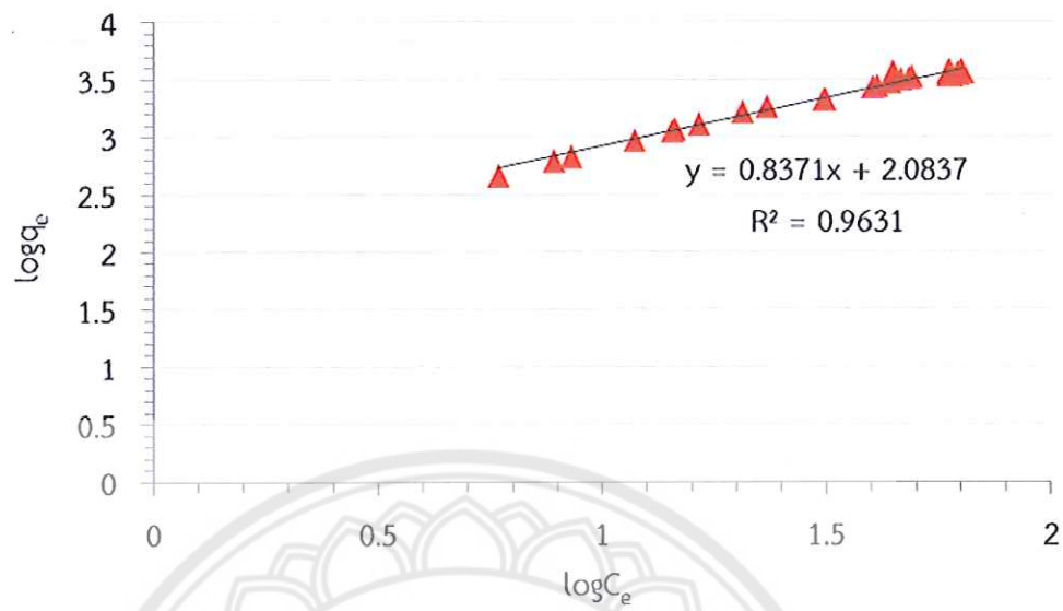
รูปที่ ๓.3 แสดงผลของสมการไอโซเทอรั่มฟรอนด์ลิชของขนาดของตัวดูดซับ 40 mesh ความสูงของตัวดูดซับ 5 เซนติเมตร อัตราการไหล 5 มิลลิลิตรต่อนาที และความเข้มข้นเริ่มต้นของสารละลายสีย้อมเมทิลีนบลู 50 มิลลิกรัมต่อลิตร
