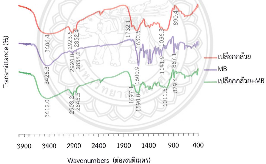
รูปที่ 4.2 FT-IR spectrometer แสดงลักษณะทางเคมีของเปลือกกัลวยี่ สีย้อมเมทิลีนบลู และเปลือกกัลวยี่ี่ผ่านการดูดซับเมทิลีนบลู
