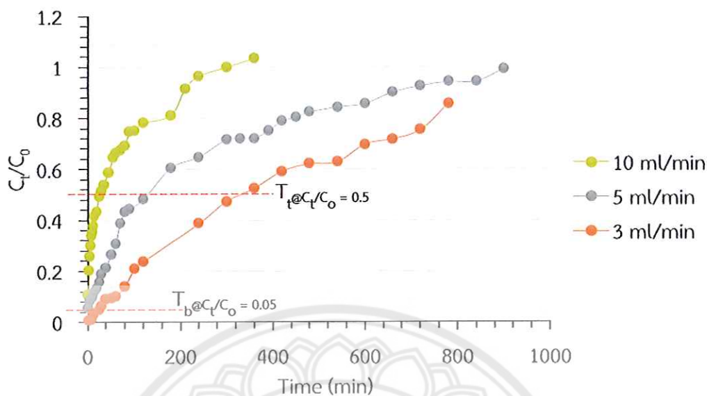
รูปที่ 4.7 แสดงความสัมพันธ์ C_t/C_0 กับเวลา ที่อัตราการไหลของสารละลายสีย้อมต่างๆ คือ 3 5 และ 10 มิลลิลิตรต่อนาที ขนาดของตัวดูดซับ 12 เมช ความสูง 5 เซนติเมตร และความเข้มข้นเริ่มต้นของสารละลายสีย้อมเมทิลีนบลู 600 มิลลิกรัมต่อลิตร
