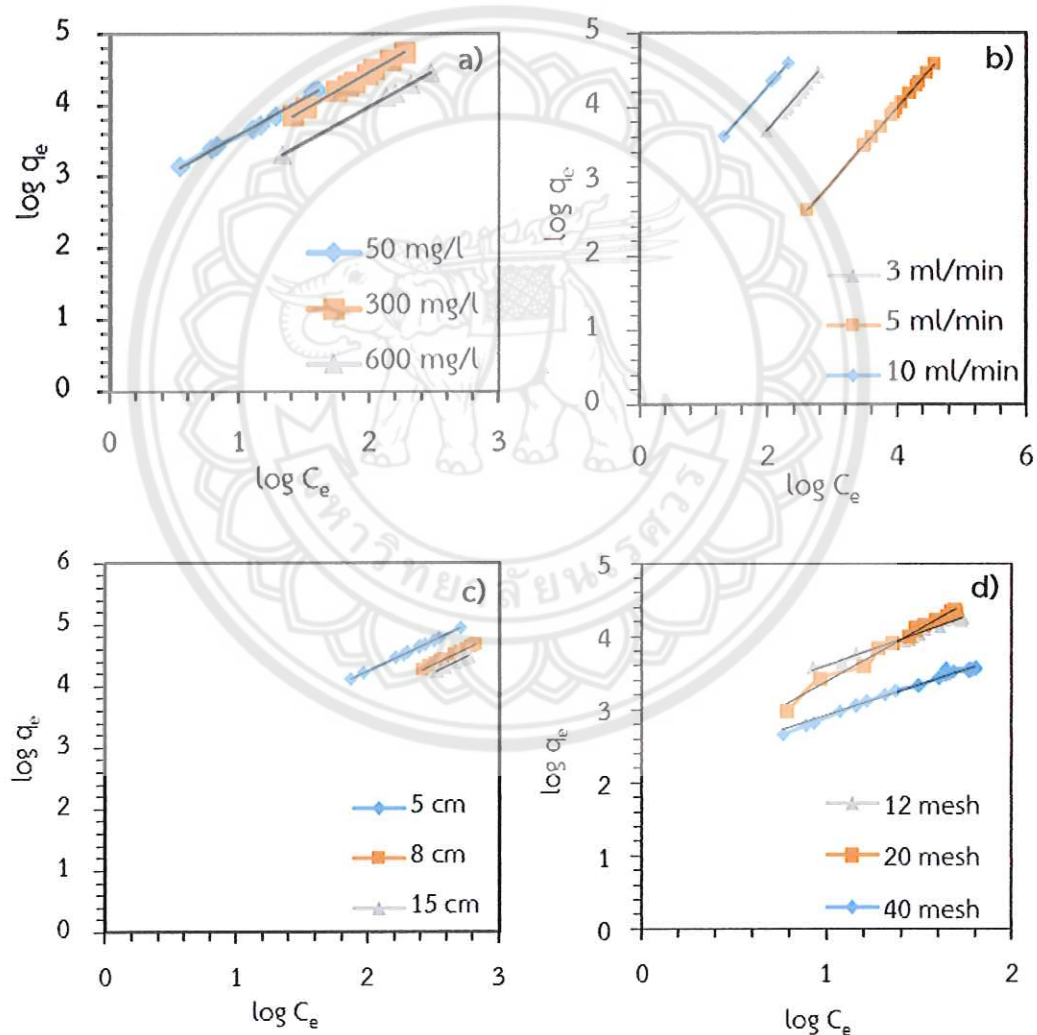
รูปที่ 4.14 สมการไอโซเทิร์มของการดูดซับฟรุนด์ลิช a) ความเข้มข้นเริ่มต้นของสีย้อมเมทิลีนบลู b) อัตราการไหลของสีย้อมเมทิลีนบลู c) ความสูงของตัวดูดซับ และ d) ขนาดของตัวดูดซับ
