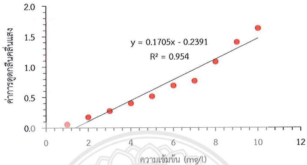
รูปที่ ๑.1 กราฟมาตรฐาน
