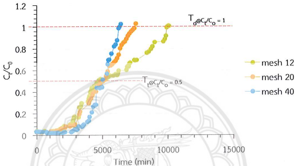
รูปที่ 4.11 แสดงความสัมพันธ์ C_t/C_0 กับเวลาที่ขนาดของตัวดูดซับ 12 20 และ 40 เมช ความสูงของตัวดูดซับ 5 เซนติเมตร อัตราการไหล 5 มิลลิลิตรต่อนาที และความเข้มข้นเริ่มต้นของสารละลายสีย้อมเมทิลีนบลู 50 มิลลิกรัมต่อลิตร
