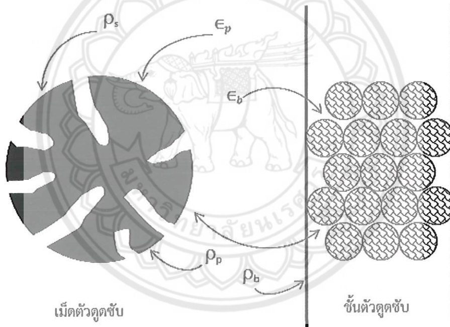
รูปที่ 2.5 ความหนาแน่นประเภทต่างๆ ของระบบดูดซับ ช่องว่างในเม็ดตัวดูดซับและระหว่างเม็ดตัวดูดซับ [4]
