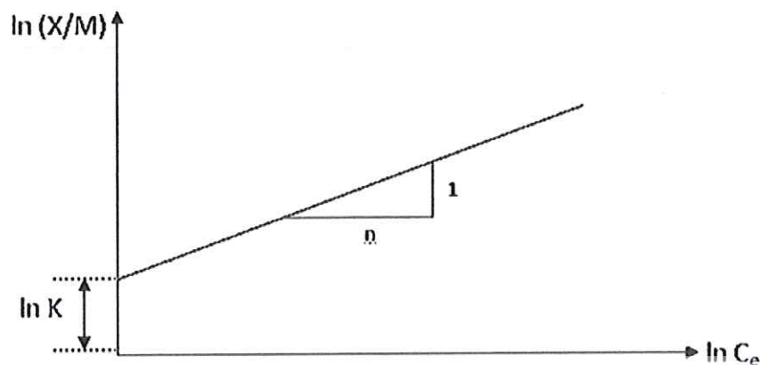
รูปที่ 2.3 กราฟแสดงความสัมพันธ์ระหว่าง \ln(X/M) และ \ln C_e [14]
