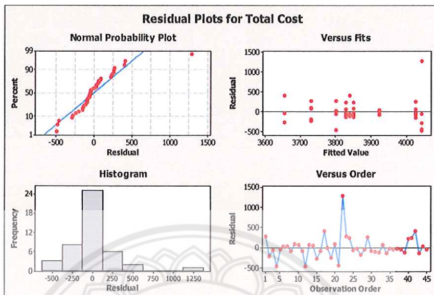
รูปที่ 4.33 แสดงการวิเคราะห์ ANOVA ของปัญหาขนาดกลางที่ 1
