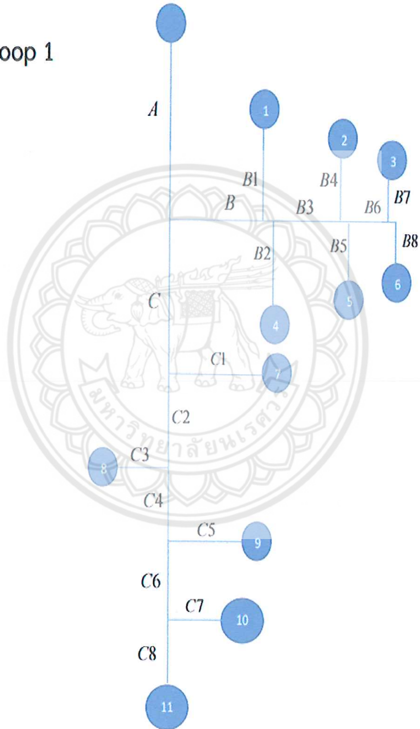
รูปที่ 3.2 ภาพไดอะแกรมระบบท่อ loop 1
