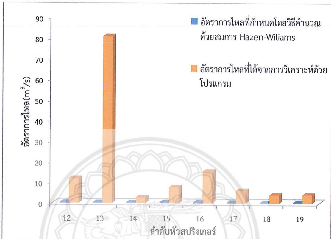
รูปที่ 4.17 แผนภูมิแสดงการเปรียบเทียบอัตราการไหล loop ที่ 2
