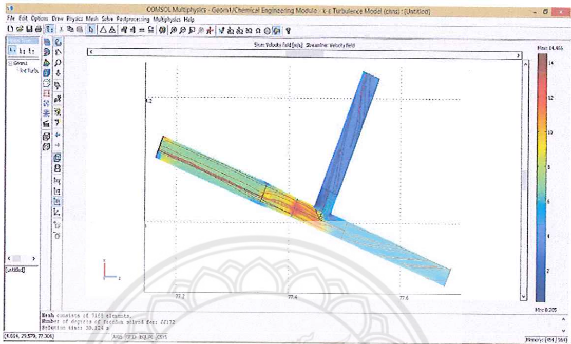
รูปที่ ง.6 ผลจากการวิเคราะห์ของโปรแกรม Comsol Multiphysics™
