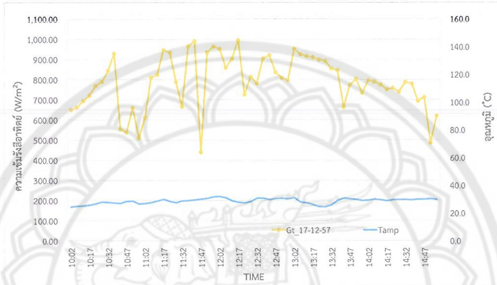
รูปที่ 31 ค่าความเข้มรังสีอาทิตย์และอุณหภูมิแวดล้อมเฉลี่ย วันที่ 17 ธันวาคม 2557
