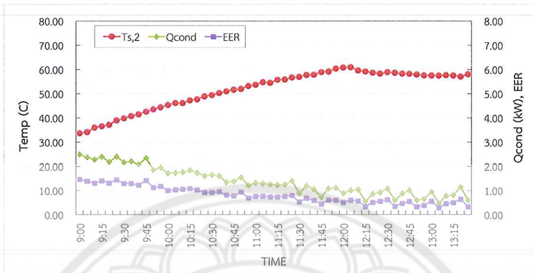
รูปที่ 34 ความสัมพันธ์อุณหภูมิน้ำถังที่ 2 ( T_{s2} ), Q_{Cond} และ EER ของระบบผลิตน้ำร้อนจากปั๊มความร้อน เมื่อควบคุมอุณหภูมิน้ำในถังที่ 1 ที่ 30^{\circ}\text{C} (วันที่ 24 ธันวาคม 2557)
