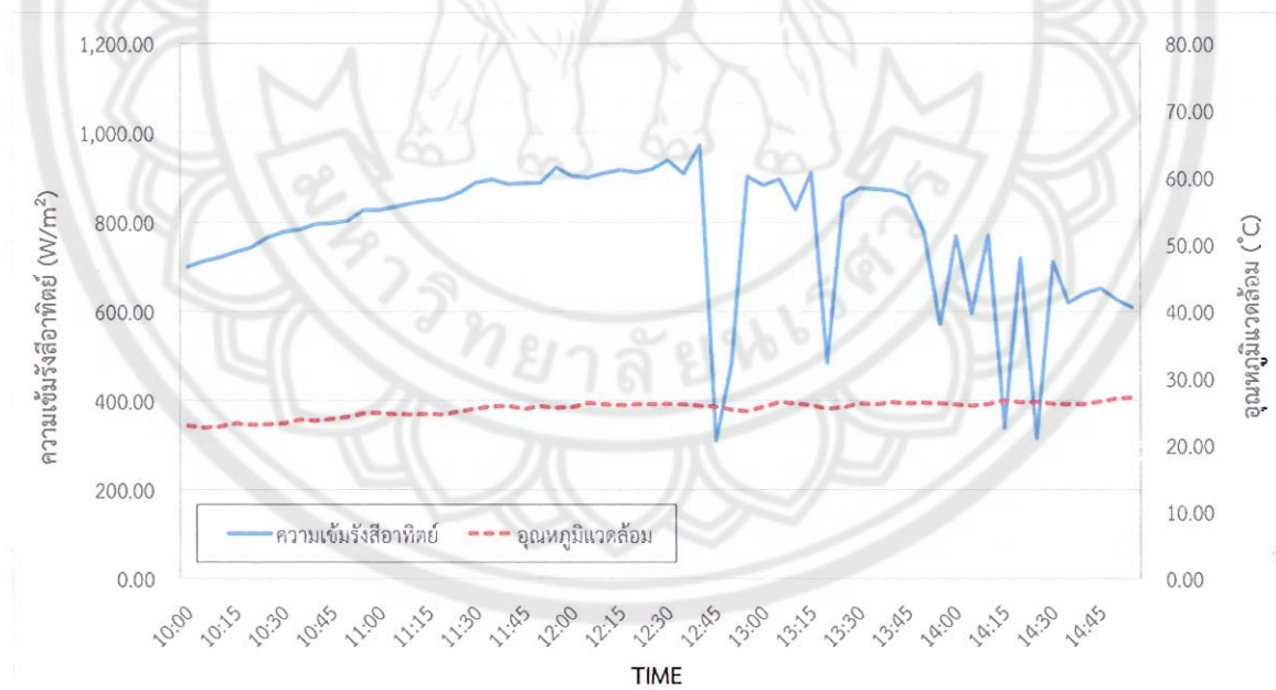
รูปที่ 26 ค่าความเข้มรังสีอาทิตย์และอุณหภูมิแวดล้อมเฉลี่ย วันที่ 21 ธันวาคม 2557
