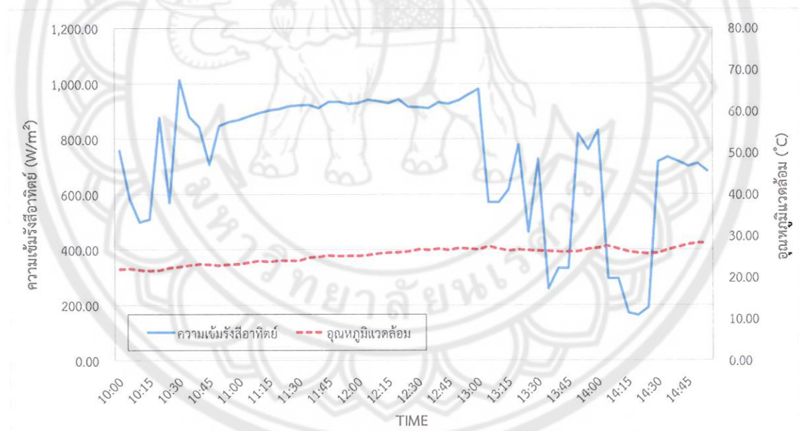
รูปที่ 24 ค่าความเข้มรังสีอาทิตย์และอุณหภูมิแวดล้อมเฉลี่ย วันที่ 20 ธันวาคม 2557
