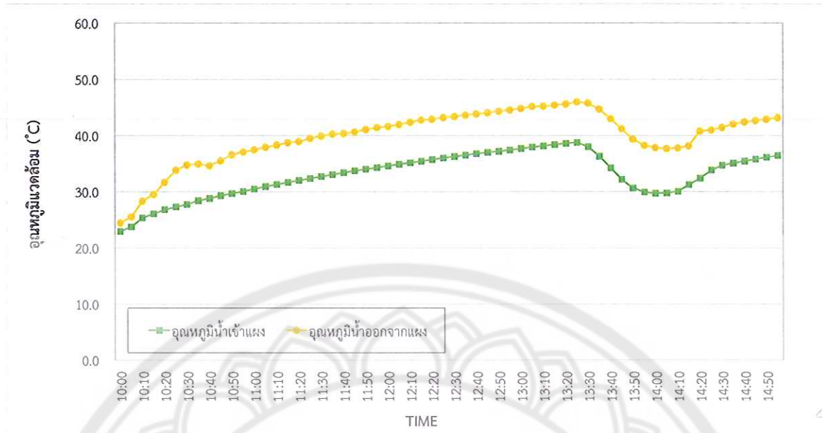
รูปที่ 25 อุณหภูมิน้ำเข้าและน้ำออกจากแผงเซลล์แสงอาทิตย์ วันที่ 20 ธันวาคม 2557
