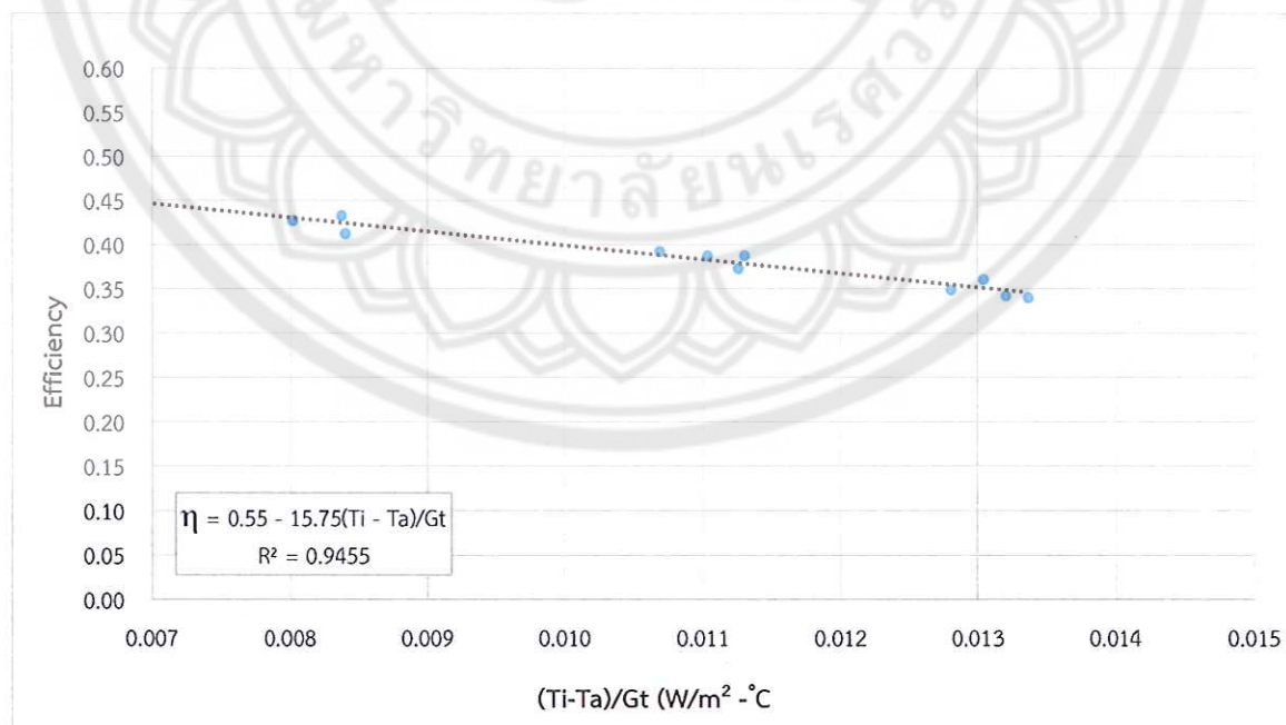
รูปที่ 30 สมรรถนะทางความร้อนของระบบผลิตน้ำร้อนที่ได้จากลมร้อนที่ระบายออกจากหลังแผงเซลล์แสงอาทิตย์
