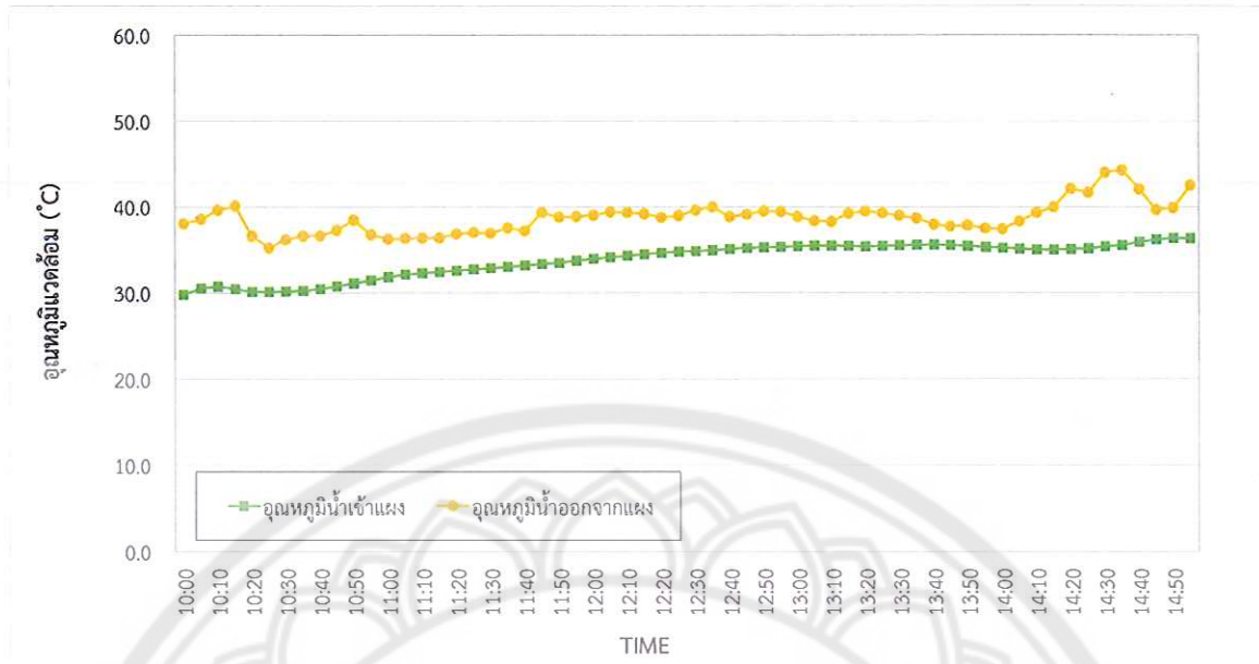
รูปที่ 27 อุณหภูมิน้ำเข้าและน้ำออกจากแผงเซลล์แสงอาทิตย์ วันที่ 21 ธันวาคม 2557
