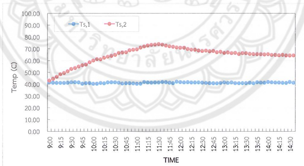
รูปที่ 35 ความสัมพันธ์อุณหภูมิน้ำถังที่ 1 ( T_{s1} ) และอุณหภูมิน้ำถังที่ 2 ( T_{s2} ) ของระบบผลิตน้ำร้อนจากปั๊มความร้อน เมื่อควบคุมอุณหภูมิน้ำในถังที่ 1 ที่ 40^{\circ}\text{C} (วันที่ 26 ธันวาคม 2557)
