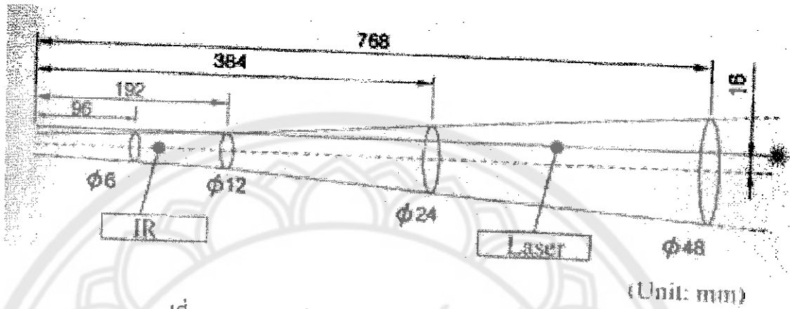
รูปที่ 7.2 ระยะการทำงานของ Infrared Thermometer ST-8828
