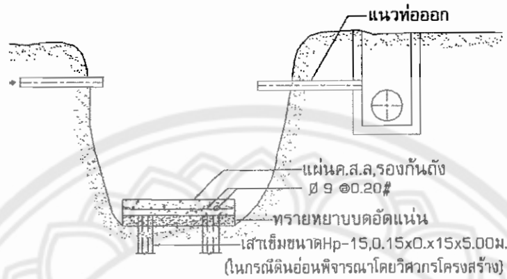
รูปที่ ผนวก ข.2 การติดตั้งถังบำบัดน้ำเสีย บริษัท B ขั้นตอนที่ 1
