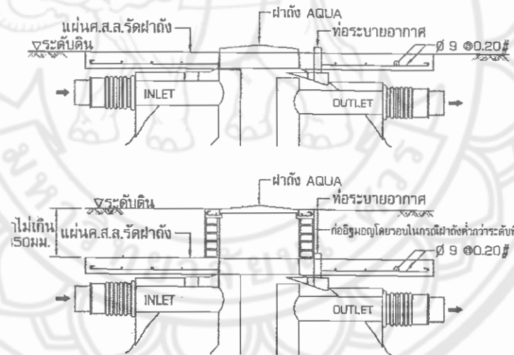
รูปที่ ผนวก ข.7 การติดตั้งถังบำบัดน้ำเสีย บริษัท B ชั้นตอนที่ 6
