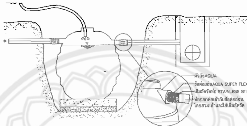
รูปที่ ผนวก ข.4 การติดตั้งถังบำบัดน้ำเสีย บริษัท B ชั้นตอนที่ 3
