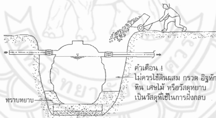
รูปที่ ผนวก ข.5 การติดตั้งถังบำบัดน้ำเสีย บริษัท B ชั้นตอนที่ 4
