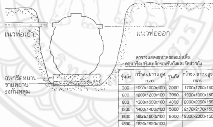
รูปที่ ผนวก ข.3 การติดตั้งถังบำบัดน้ำเสีย บริษัท B ขั้นตอนที่ 2
