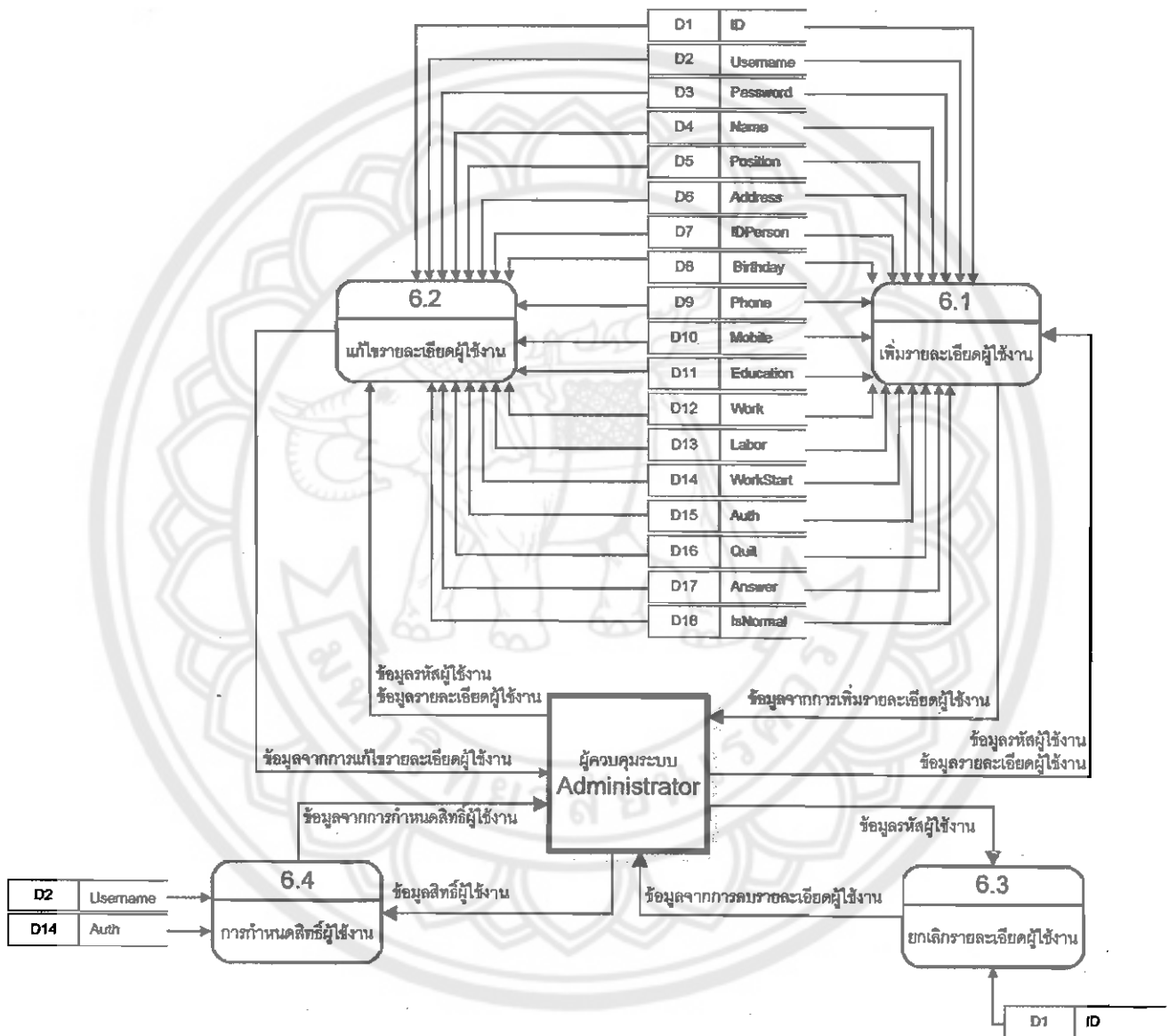
รูปที่ 4.4 โครงสร้างส่วน Data Flow Diagram level 2 ผู้ควบคุมระบบ (1)
