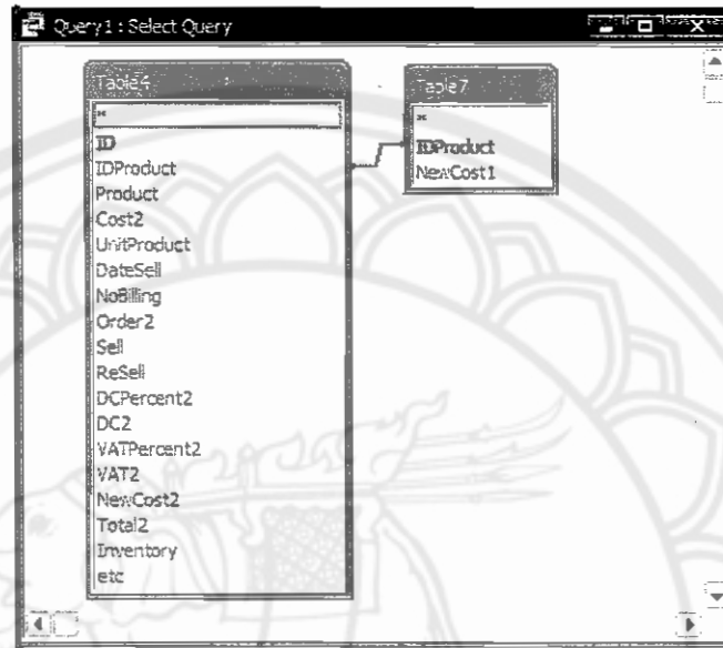
รูปที่ 4.19 ชนิดของข้อมูลและความสัมพันธ์ของ Query1
