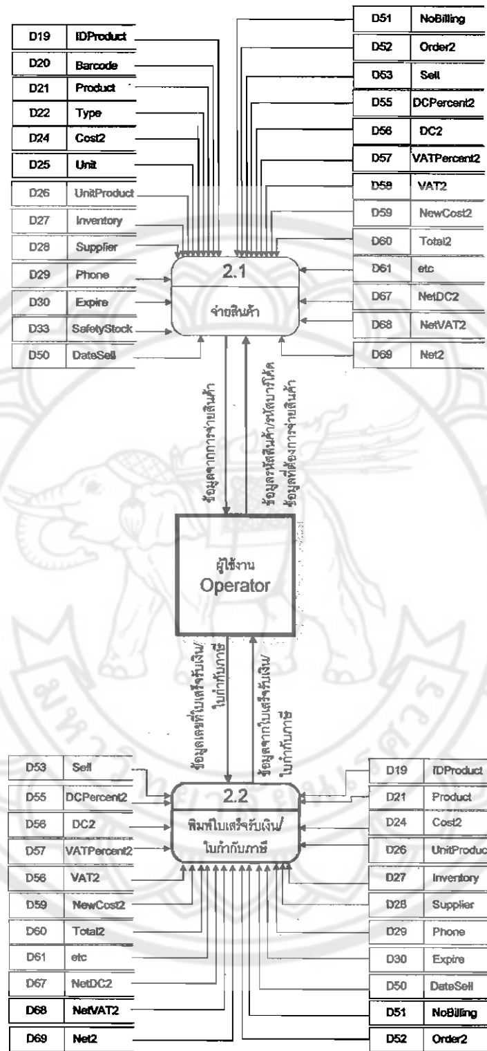
รูปที่ 4.10 โครงสร้างส่วน Data Flow Diagram level 2 ผู้ใช้งาน (2)
