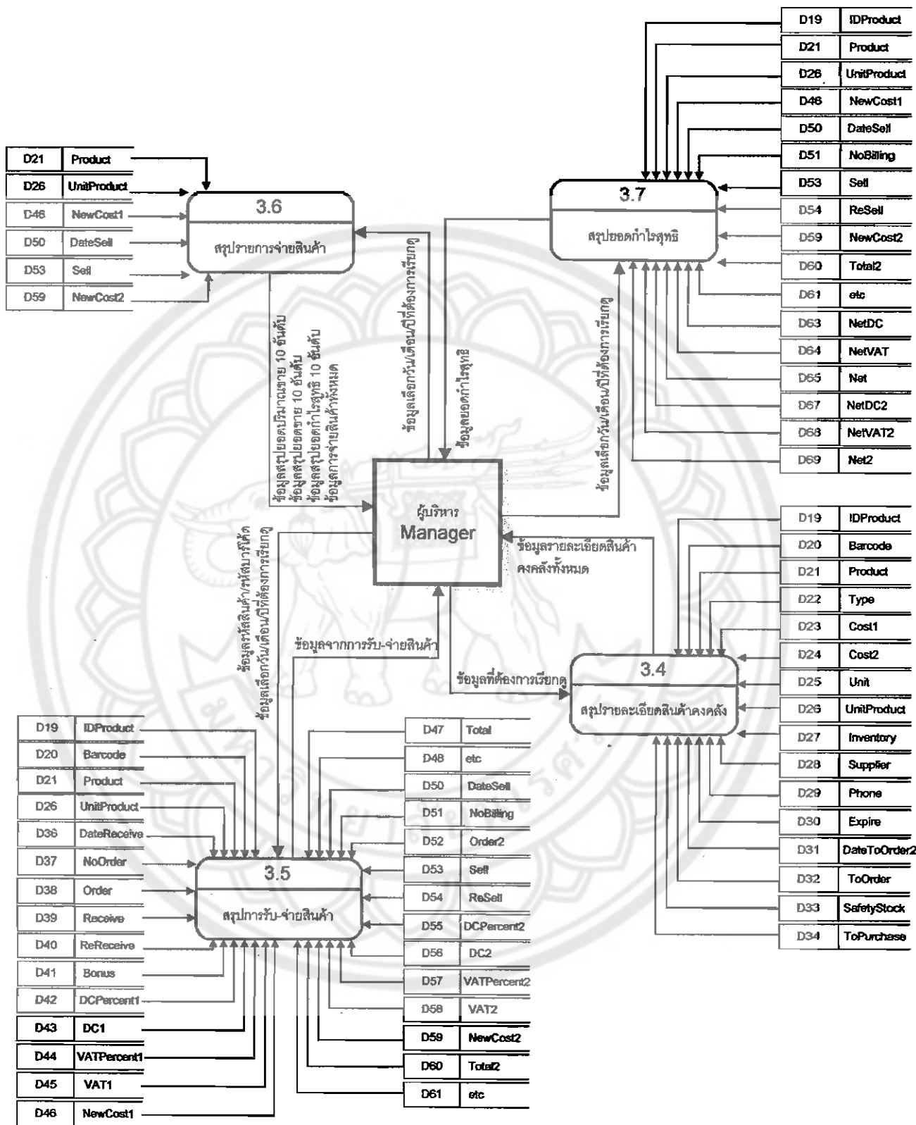
รูปที่ 4.6 โครงสร้างส่วน Data Flow Diagram level 2 ผู้บริหาร (1)
