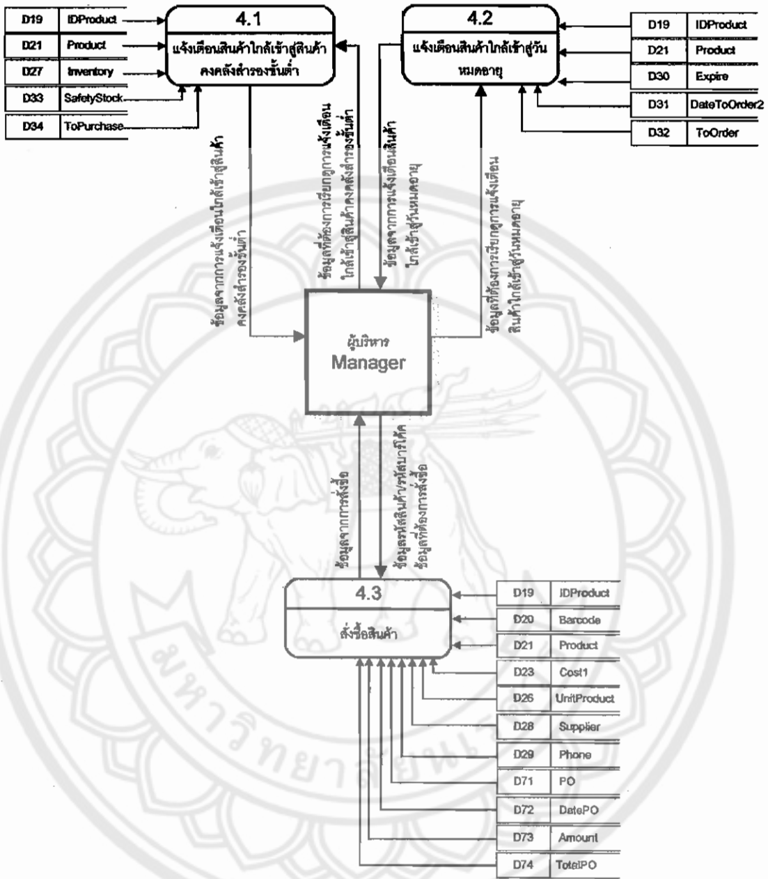
รูปที่ 4.7 โครงสร้างส่วน Data Flow Diagram level 2 ผู้บริหาร (2)
