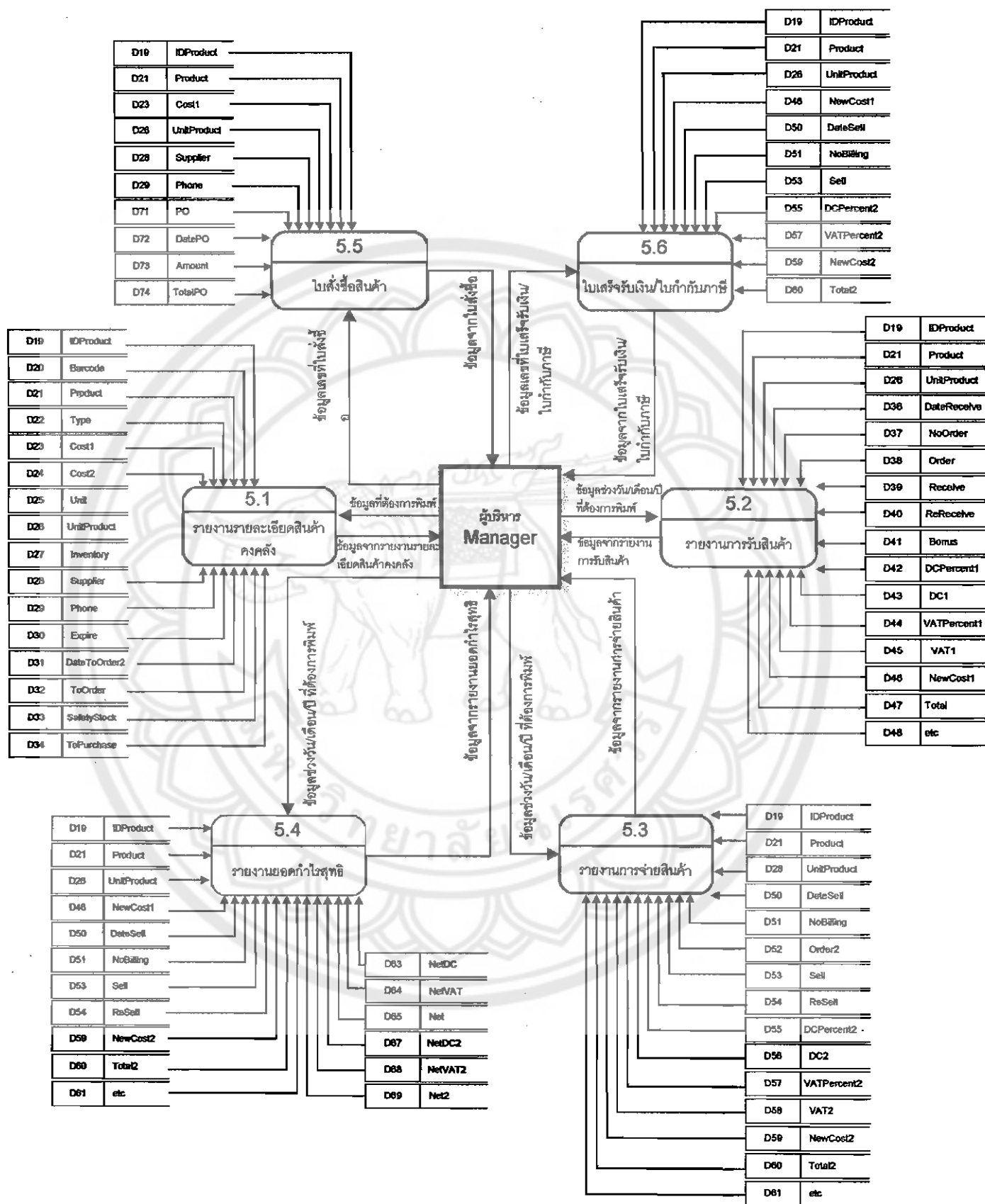
รูปที่ 4.8 โครงสร้างส่วน Data Flow Diagram level 2 ผู้บริหาร (3)
