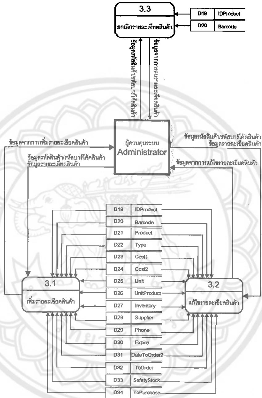
รูปที่ 4.5 โครงสร้างส่วน Data Flow Diagram level 2 ผู้ควบคุมระบบ (2)
