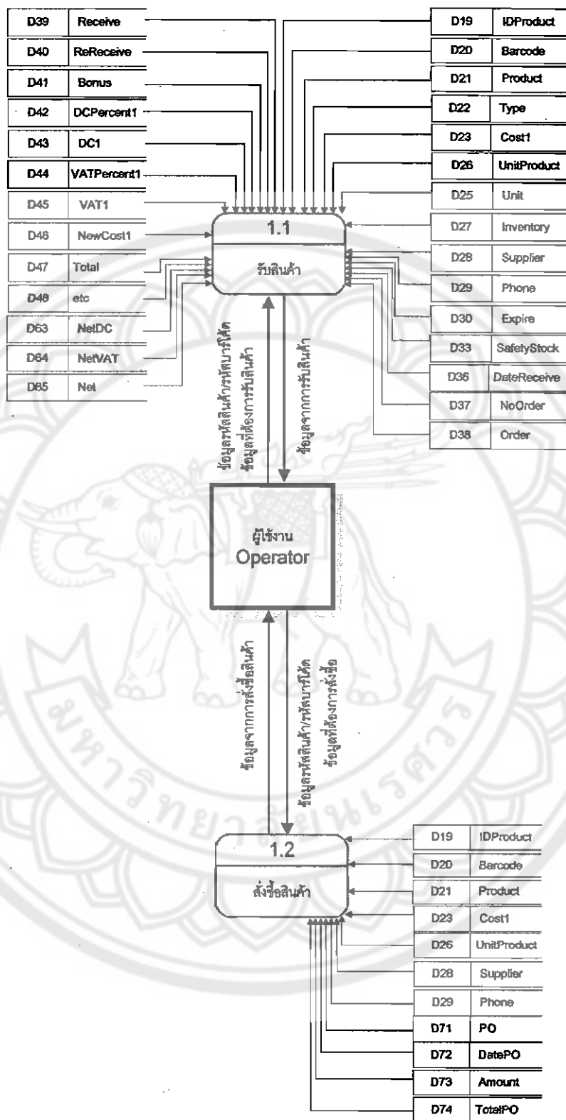
รูปที่ 4.9 โครงสร้างส่วน Data Flow Diagram level 2 ผู้ใช้งาน (1)
