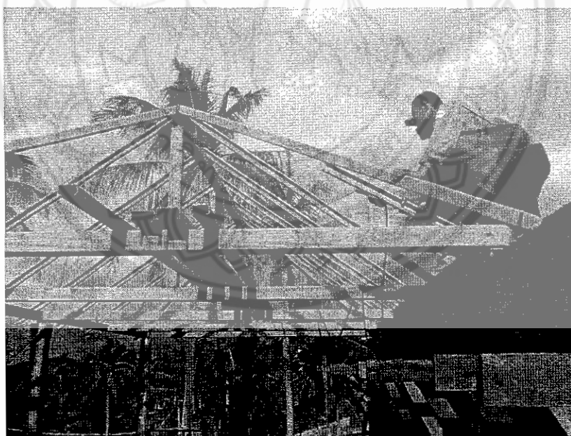
รูปที่ 8 แสดงงานติดตั้งจันทันย่อย
