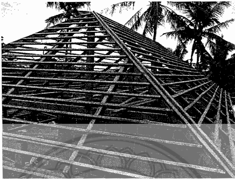
รูปที่13 แสดงงานติดตั้งแปหลังคาขึ้นบนสำเร็จ
