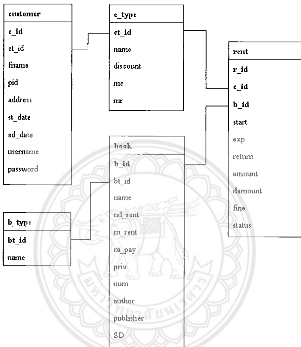
รูปที่ 3.8 ความสัมพันธ์ของตาราง
