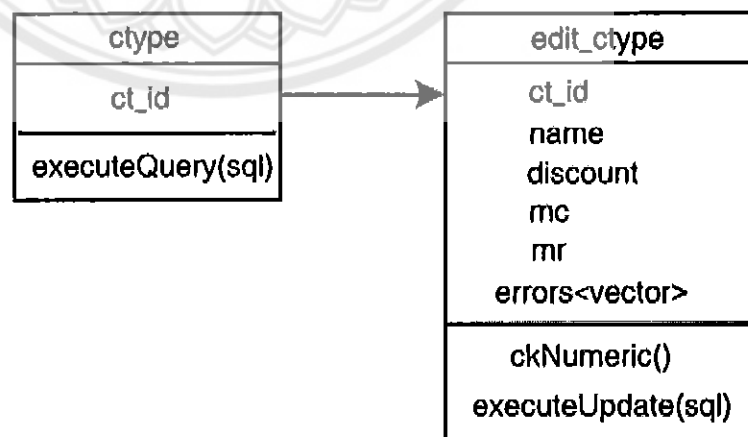
รูปที่ 3.14 Class Diagram : Customer type
