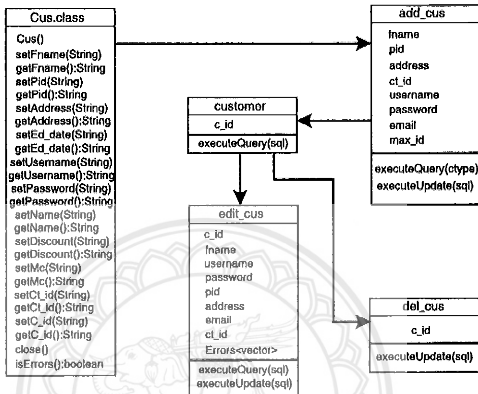
รูปที่ 3.13 Class Diagram : Customer management
