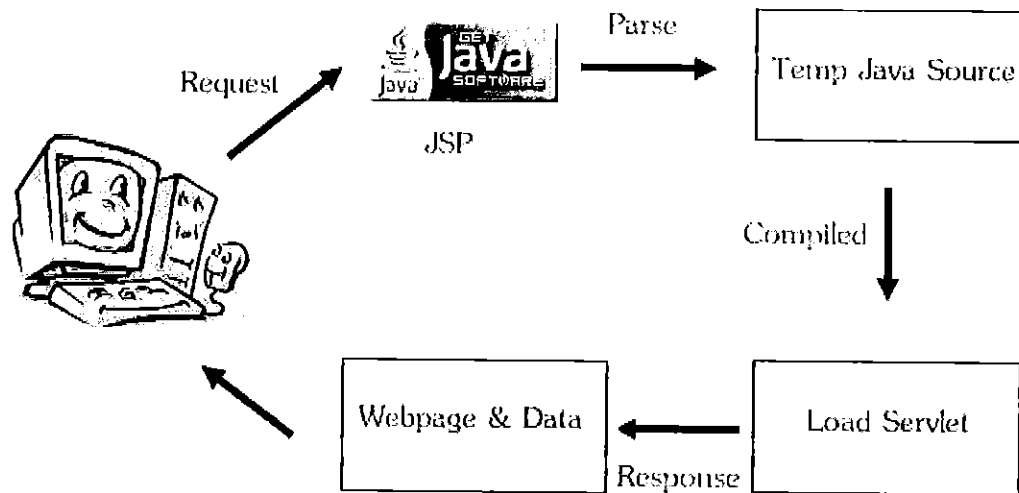
รูปที่ 2.2 การทำงานของ JSP [www.zdnet.co.uk]
