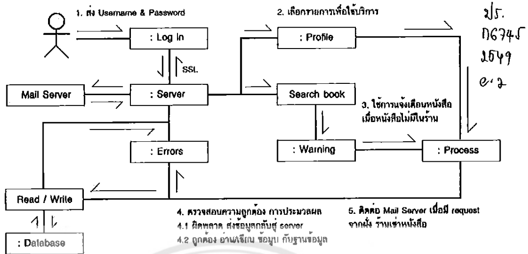
รูปที่ 3.17 Collaboration Diagram : Custome management
