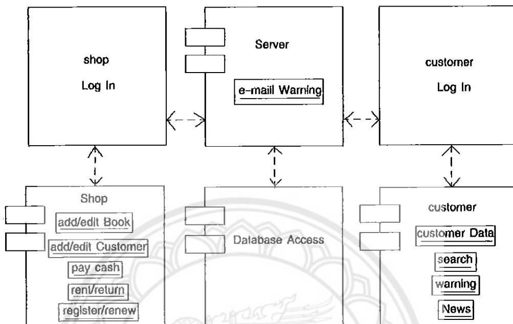
รูปที่ 3.10 Component Diagram
