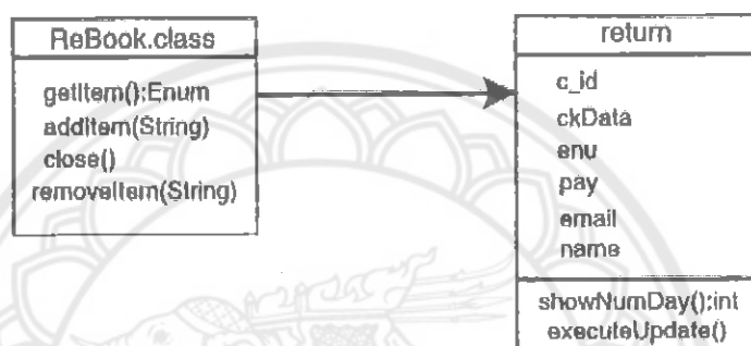
รูปที่ 3.15 Class Diagram : Rent & Return
