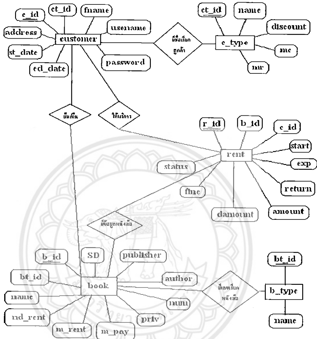
รูปที่ 3.2 ER Diagram ของฐานข้อมูลร้านหนังสือเช่า
