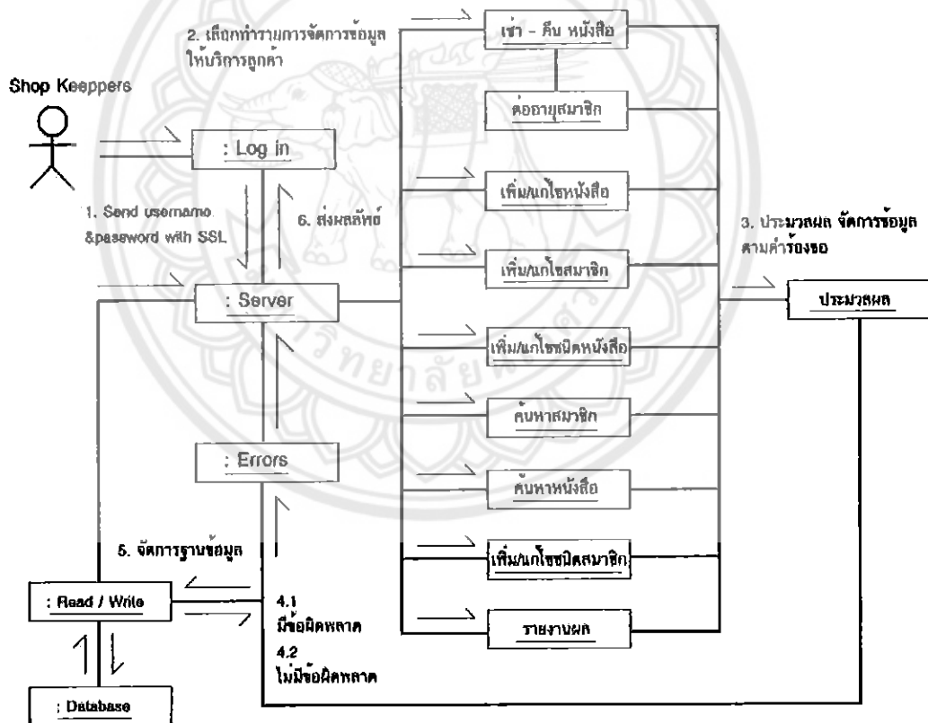
รูปที่ 3.16 Collaboration Diagram : Shop management
